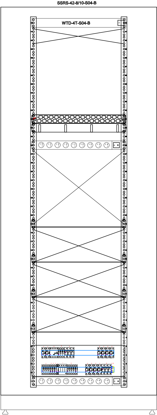
PANEL WENTYLACYJNY 4-WENTYLATOROWY DACHOWO-PODŁOGOWY Z TERMOSTATEM 1HE RAL 9005; WTD-4T-S04-B
